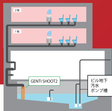
地下污水ポンプ槽 設置イメージ
